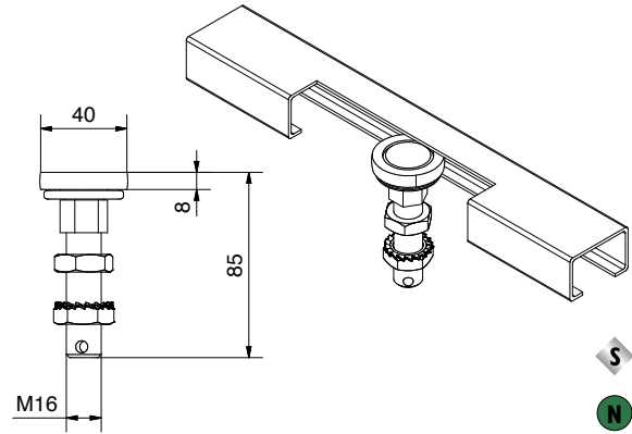
BOVENGELEIDER 104/900
