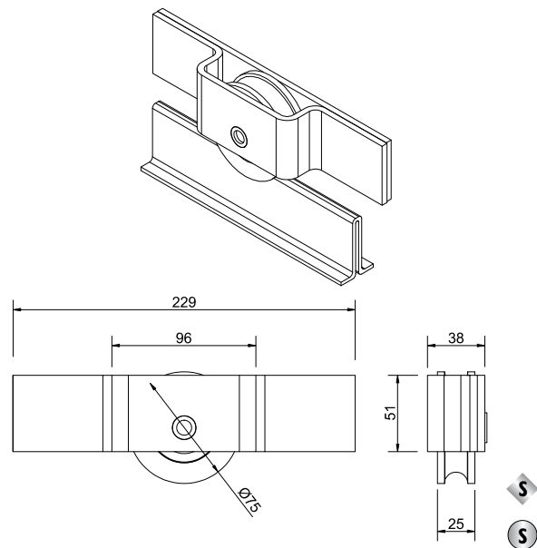
ONDERROL 5S
