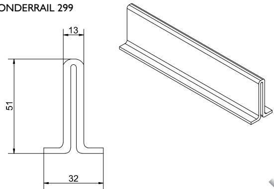
ONDERRAIL 299
