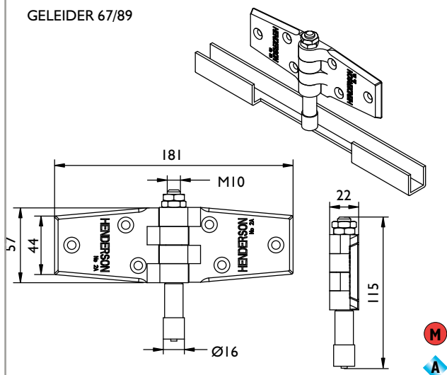
GELEIDER 67/89
