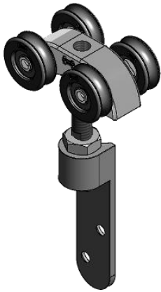
52/120/SS Hanger
