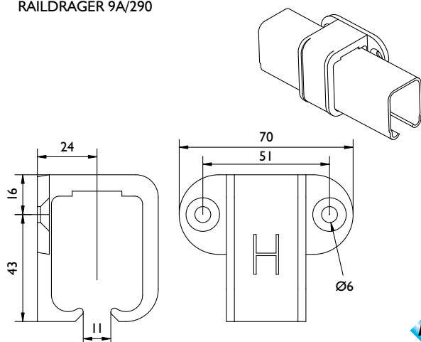
RAILDRAGER 9A/290
