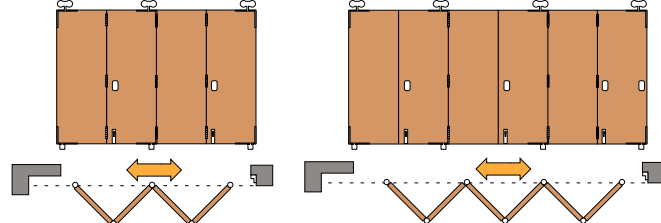
losschuivend
